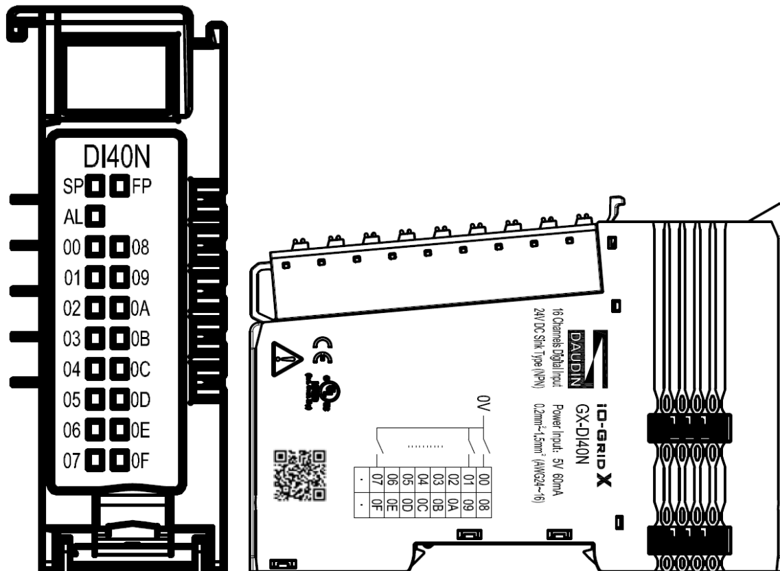
圖 4.4 GX-DI40N 圖面
